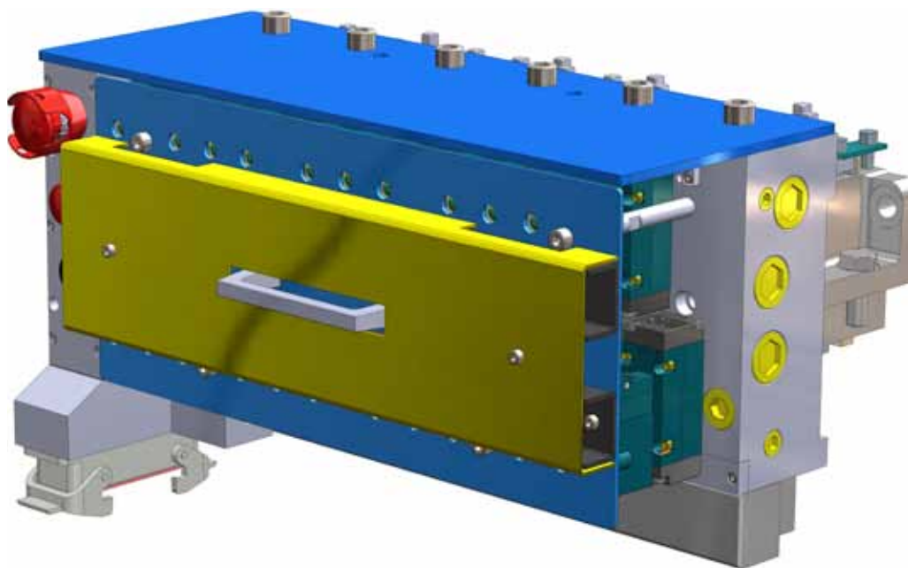
Nouveau bloc MAC Valves 21 pistes assemblé
